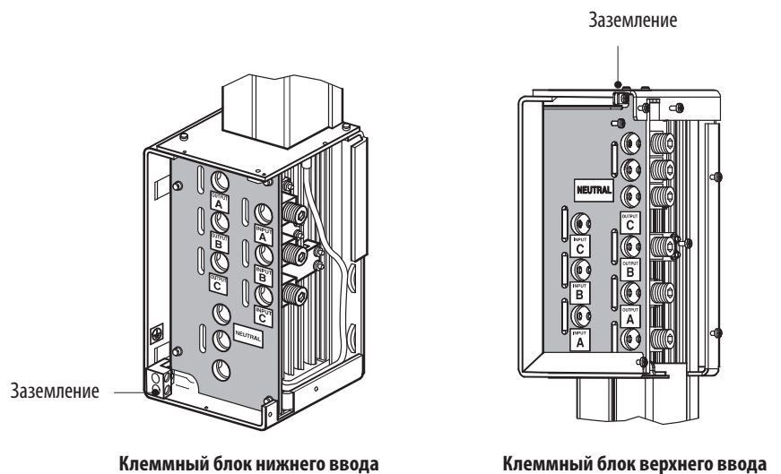
Рисунок 8. Клеммный блок шины BladeUPS
