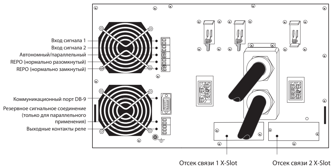
Рисунок 47. Коммуникационные опции и управляющие выходы (изображен автономный ИБП)
