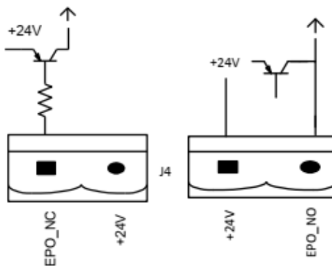
Рис. 2-23 Схема разъема системы экстренного отключения (EPO)
