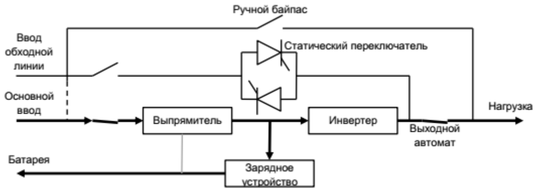
Рис. 1-3 Нормальный режим работы
