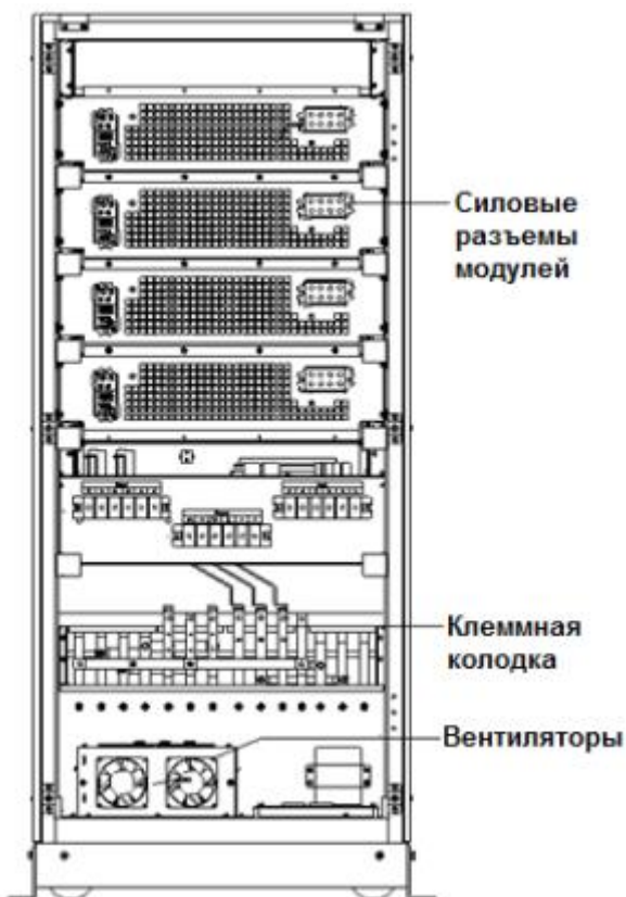
Рис. 1-11 Компоновка ИБП 80-120кВА Вид сзади
