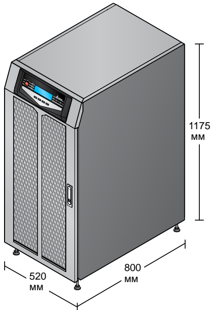
Рис. 3-1. Внешний вид и размеры ИБП 60/80 кВА
